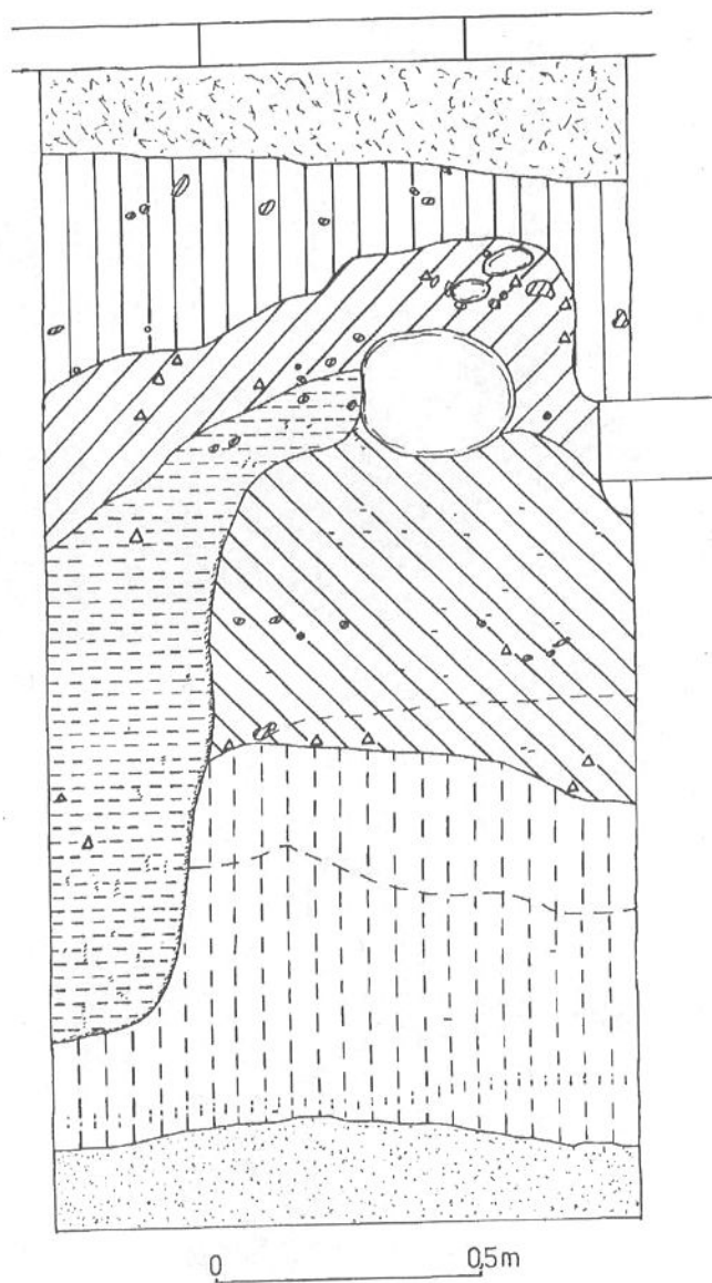
Ryc. 8. Zielona Góra, ul. Pod Filarami, wykop 1. Profil S wykopu pod studzienkę kanalizacyjną. Przekrój fragmentu dołu na wapno oraz ślady wkopów nowożytnych. W dolnej partii przekrój warstwy średniowiecznej? Rys. K. Garbacz
