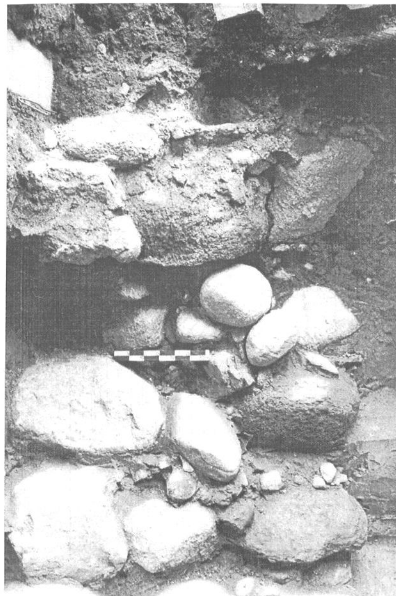
Ryc. 7. Zielona Góra, ul. Pod Filarami, wykop 1. Przekrój fundamentu muru obronnego. Kamienie w dolnej partii ułożone bez zaprawy, u góry warstwa zaprawy wapiennej. Fot. K. Garbacz
