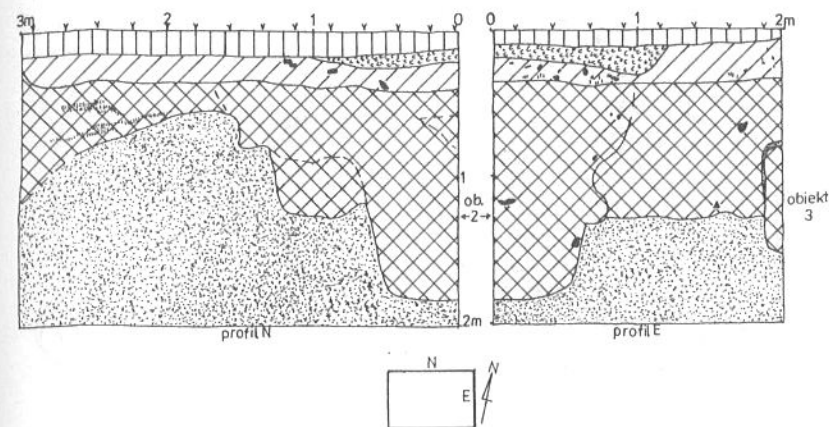
Ryc. 7. Zielona Góra, ul. Kupiecka 5-7, wykop 1. Północny i wschodni i profil
