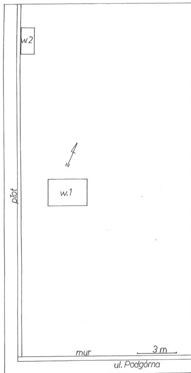
Ryc. 2. Zielona Góra. Lokalizacja wykopów przy pl. Matejki 20
